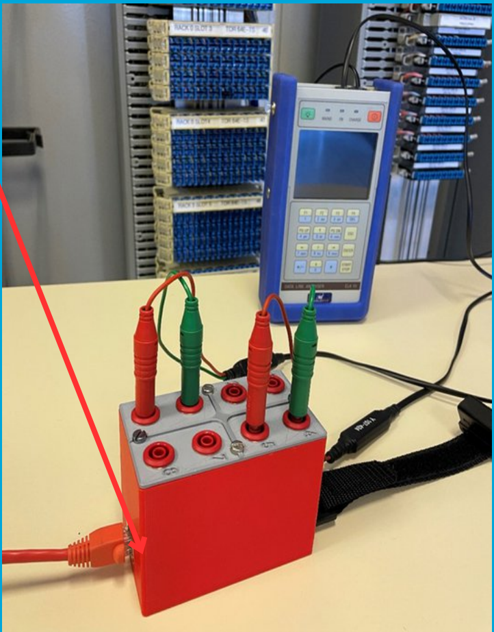
Utilisation avec un ELA10 3-6 (EM)
